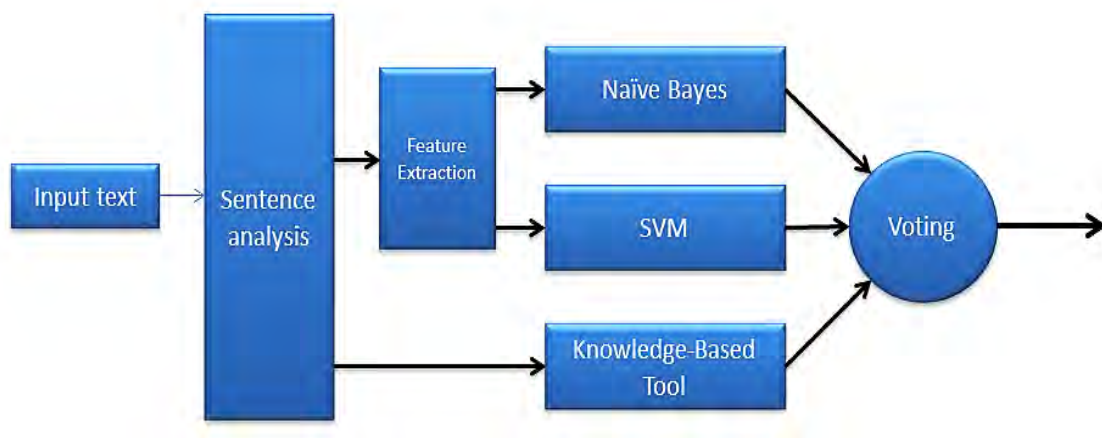
Εικόνα 5.6 Βασική αρχιτεκτονική του ομαδοποιημένου ταξινομητή.
