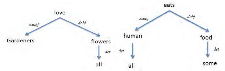
Εικόνα 3.4 Τα δέντρα Εξαρτήσεων των προτάσεων
