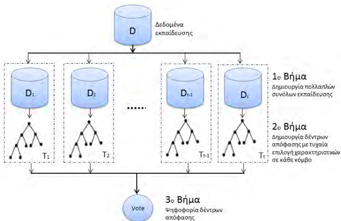
Εικόνα 6.8 Λειτουργία τυχαίων δασών.
