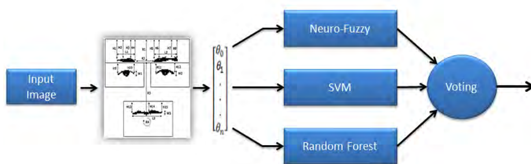
Εικόνα 6.6 Βασική αρχιτεκτονική του ομαδοποιημένου ταξινομητή.
