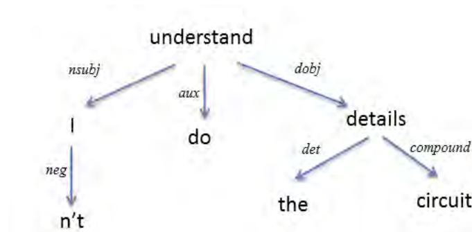
Εικόνα 4.4 Το δέντρο εξαρτήσεων της πρότασης Π2
