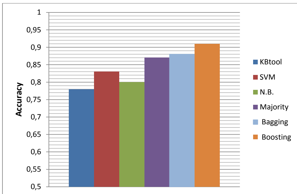
Εικόνα 5.15 Η ορθότητα των ταξινομητών σε όλο το σύνολο δεδομένων
